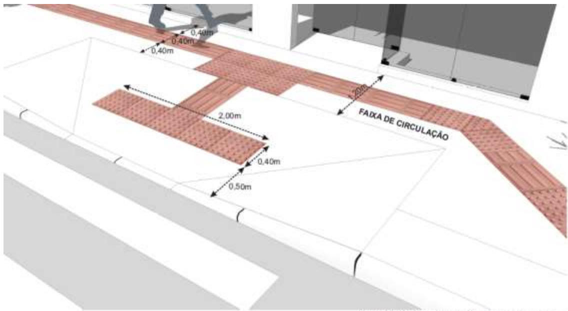
RAMPA PARA CALÇADA COM 3,00 DE LARGURA
