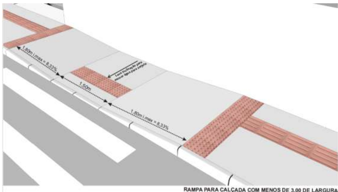
RAMPA PARA CALÇADA COM MENOS DE 3,00 DE LARGURA
